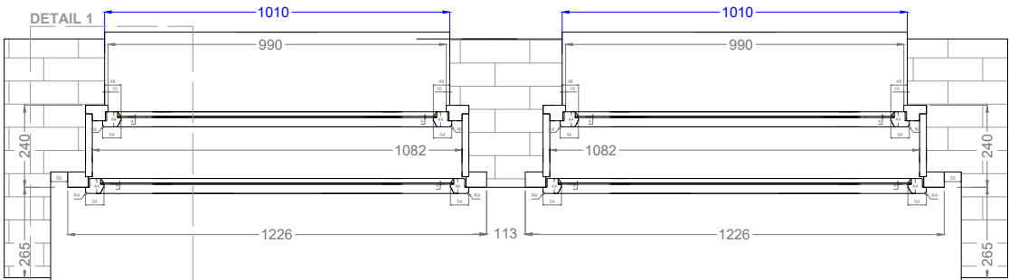
VODOROVNÝ ŘEZ B-B
