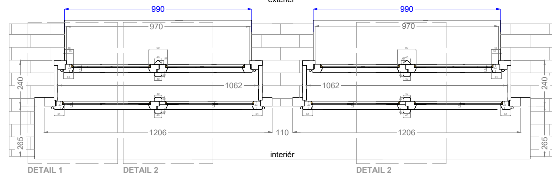
VODOROVNÝ ŘEZ A-A
