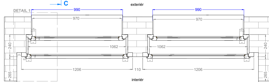
VODOROVNÝ ŘEZ B-B
