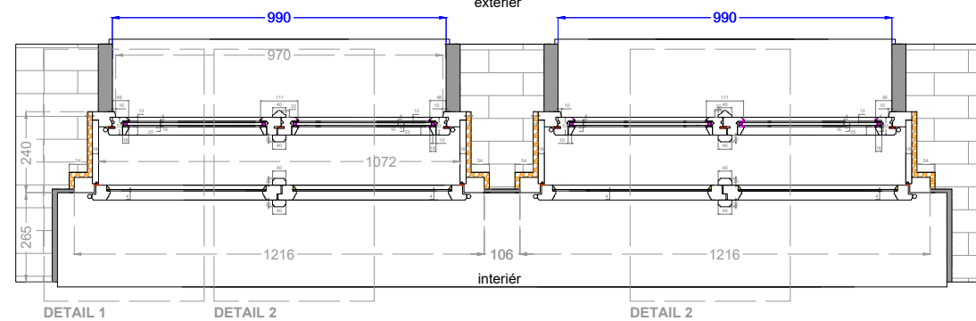
VODOROVNÝ ŘEZ D-D
