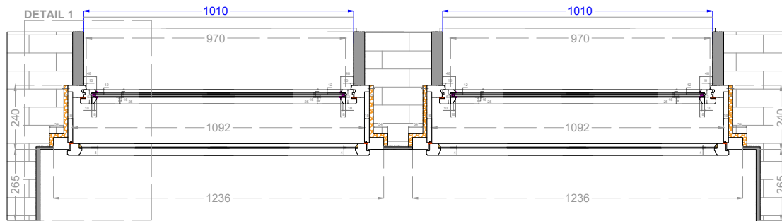
VODOROVNÝ ŘEZ E-E
