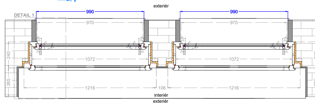
VODOROVNÝ ŘEZ E-E
