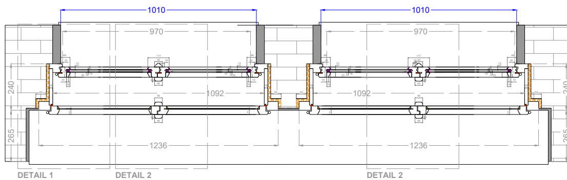
VODOROVNÝ ŘEZ D-D
