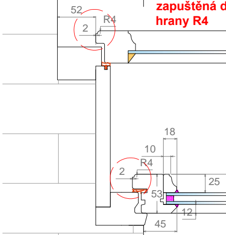
ZP4P kulatina zapuštěná R4
